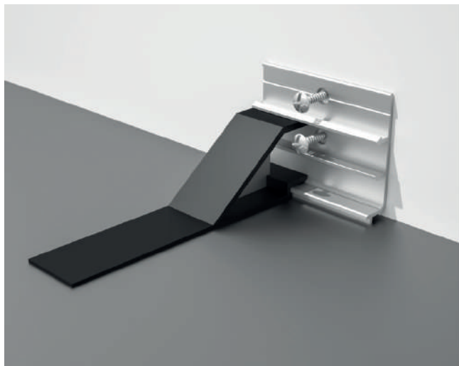
Particolare dello strumento utilizzato per posizionare in modo adeguato le guide per fissaggio battiscopa
